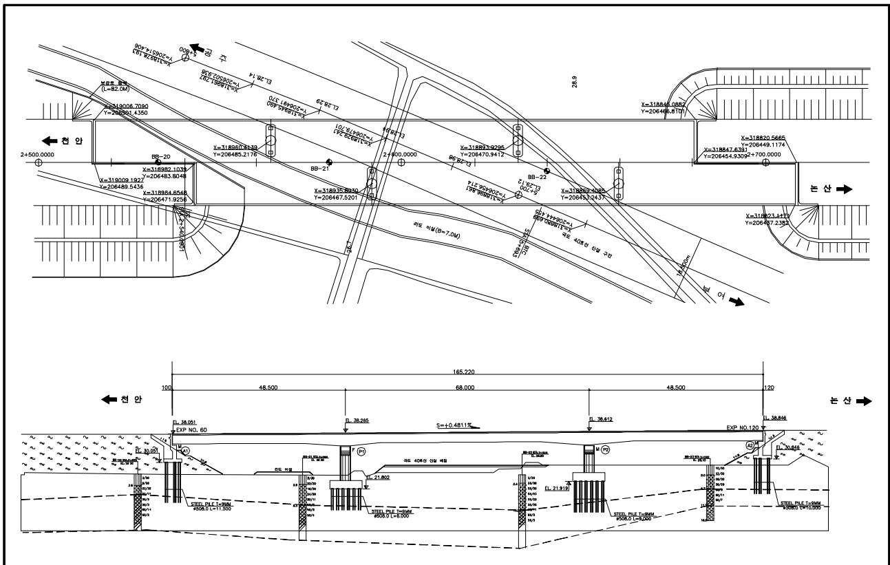
【그림 5.1】 종·평면도
